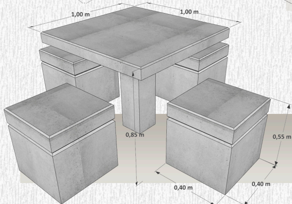
CONJUNTO MESA Y BANCO tipo dado mesa
