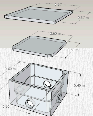
CÁMARA DE INSPECCIÓN 60 x 60cm 0,60 x 0,60 x 0,60 mts.
