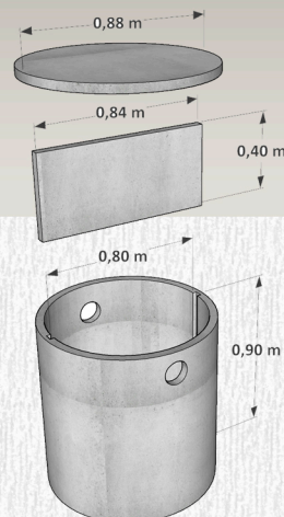
BASE CÁMARA SÉPTICA Ø800 mm Capacidad 300 Lts.
